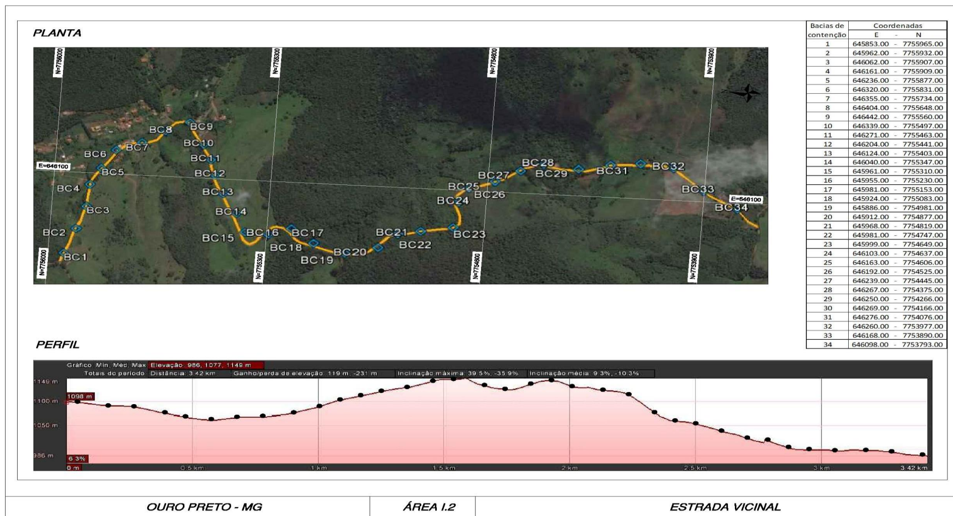
Figura 6.9 – Projeto de intervenção na estrada vicinal – Microbacia do Córrego do Andaime
