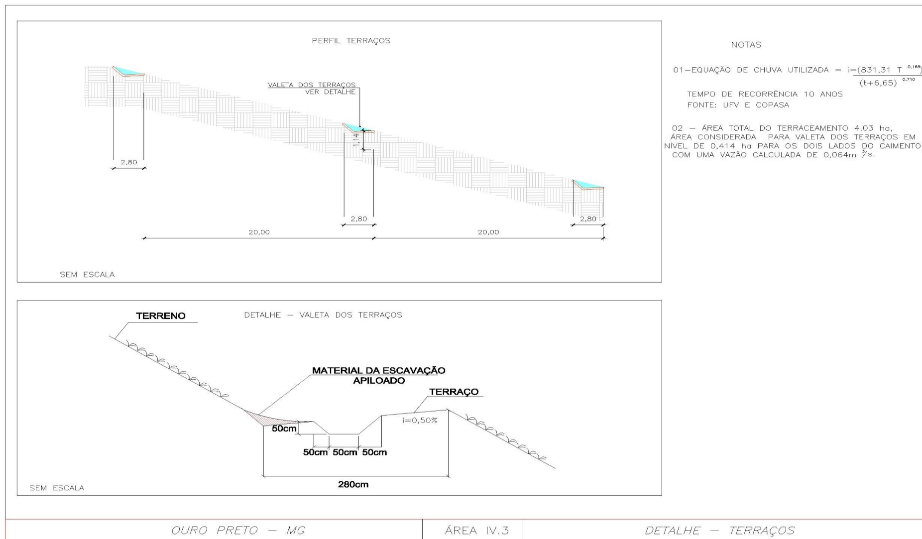
Figura 6.33 – Perfil dos terraços
