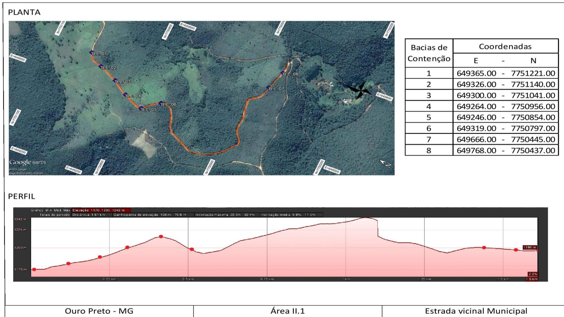
Figura 6.17 – Estrada vicinal municipal
