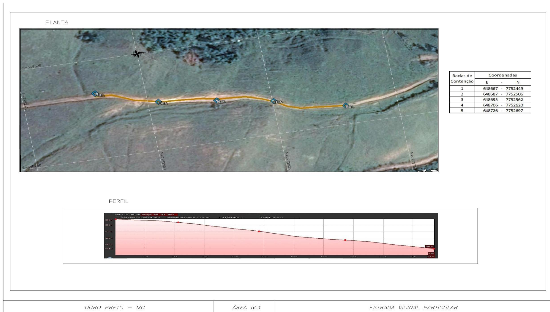
Figura 6.26 – Projeto de intervenção na estrada Vicinal – Microbacia do Córrego São Bartolomeu
