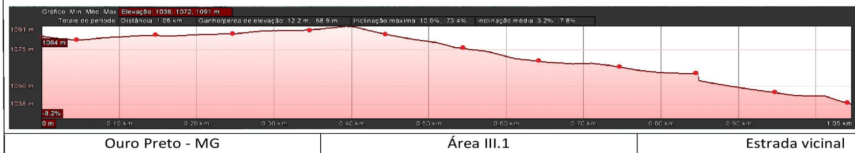
Figura 6.22 – Projeto de intervenção na estrada vicinal – Microbacia do Córrego Afogador
