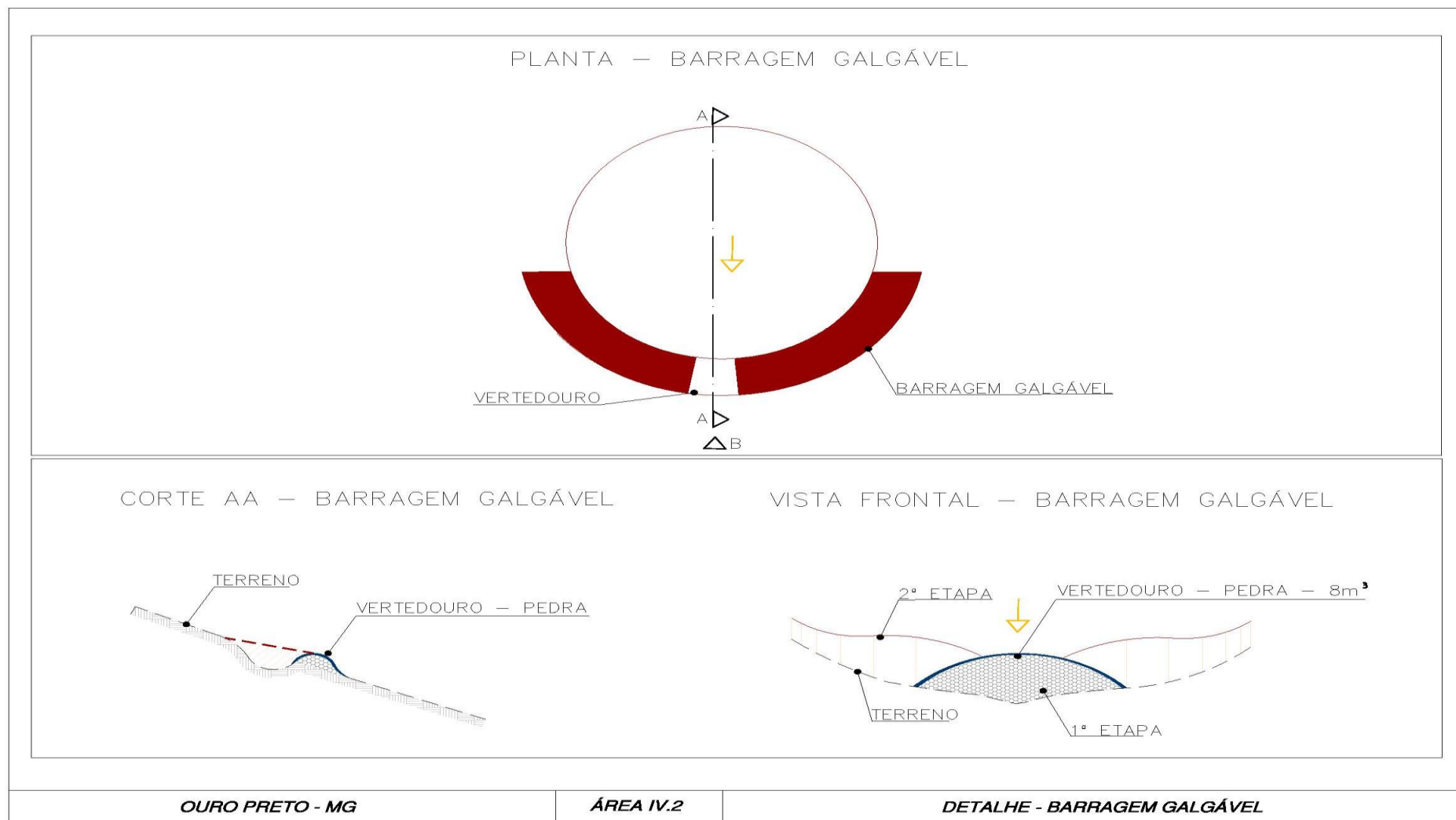
Figura 6.29 – Detalhe das barragens gálgáveis
